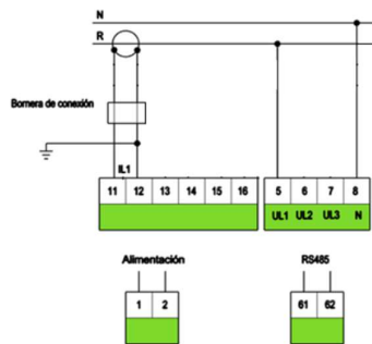
Conexión monofásica
