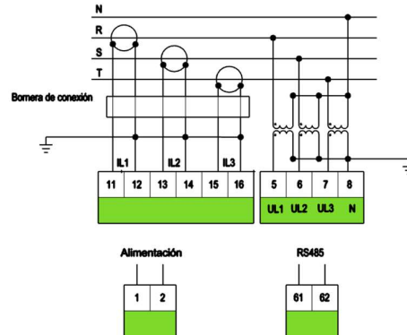
Conexión (con TC) de 4 cables con transformadores
